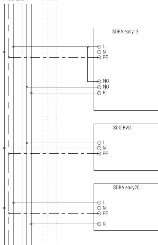
SDT-Montageschiene 7-polig N PE L1 L2 L3 + - A B C D
