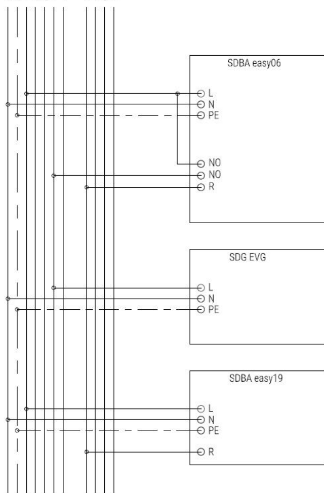
SDT-Montageschiene 11-polig N PE L1 L2 L3 + • A B C D
