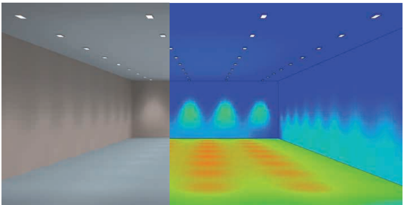
Beleuchtungsstärke (lx)
