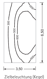
Zielbeleuchtung (Kegel)
