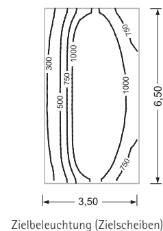
SDT + SDGOT 8000
